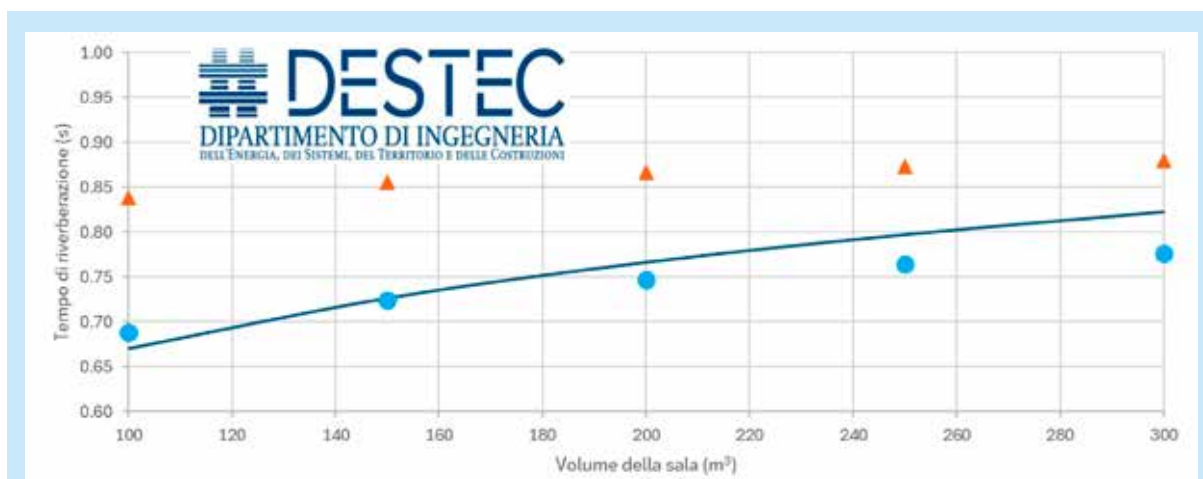
Figura: Utilità delle prestazioni acustiche del provino Bronya Light (triangoli in arancio=intonaco tradizionale, cerchi in celeste=provino ID1, linea blu= tempo di riverberazione ottimale in accordo alla normativa tecnica)
