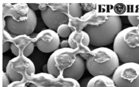
Sfere di ceramica Bronya al microscopio digitale in HD
