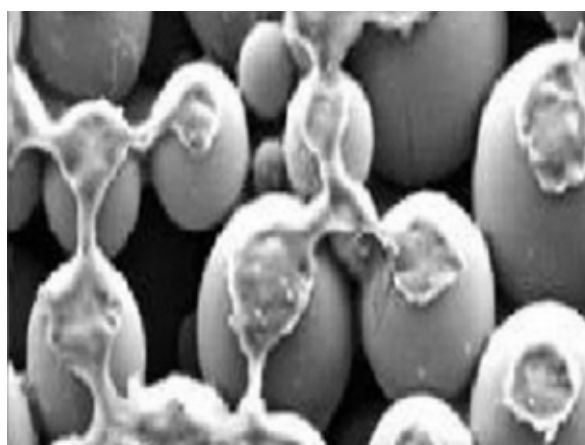
Fig. - Isolante Termico Bronya: al microscopio è visibile la speciale micro-struttura: sfere di ceramica cave legate con polimeri che impediscono il trasferimento di calore attraverso il materiale.
